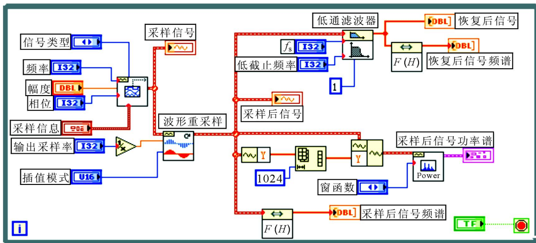
图 2 后程序框图 (The block diagram)
