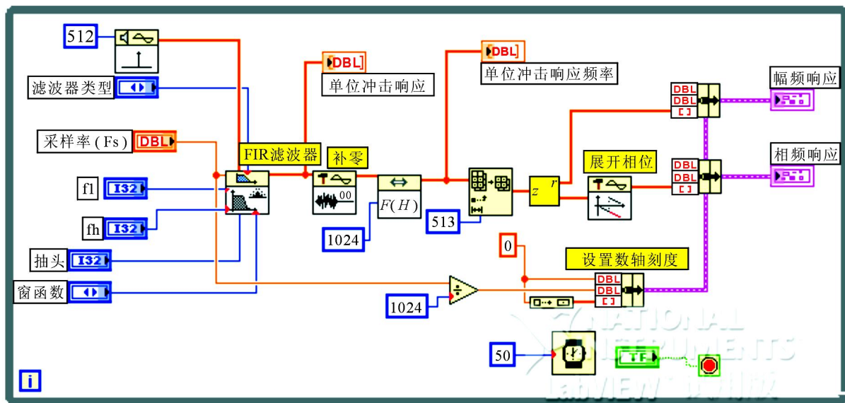
图 4 后程序框图 (The block diagram)
